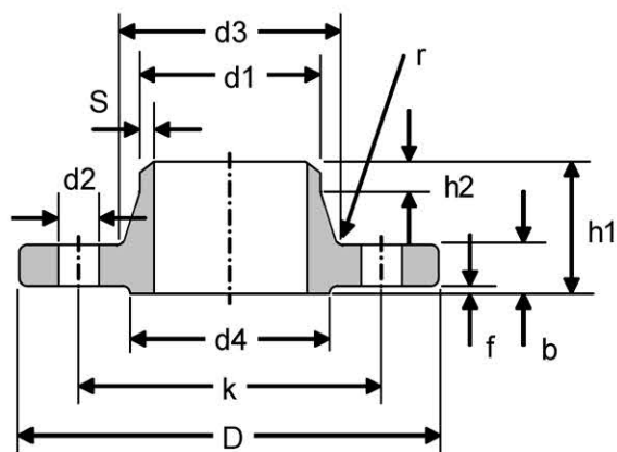
DIN 2637 PN100
