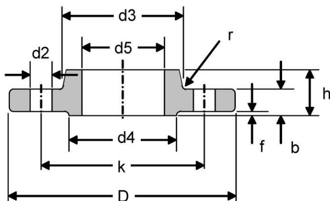
DIN86029 PN10
