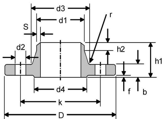
DIN2627 PN400
