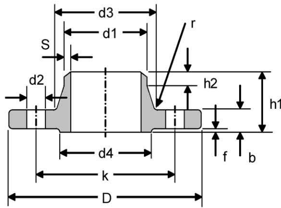
DIN 2635 PN40
