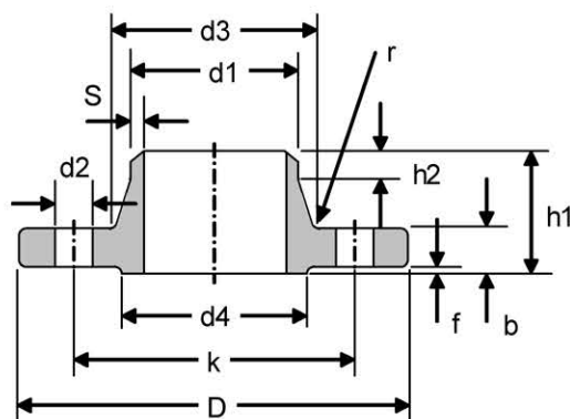
DIN2629 PN320
